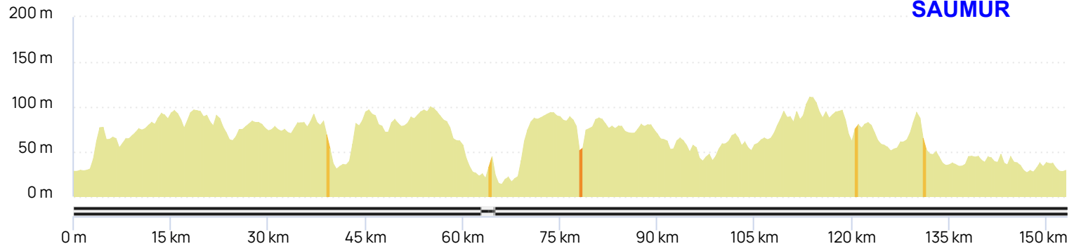
Profil en Long de l'itinéraire
